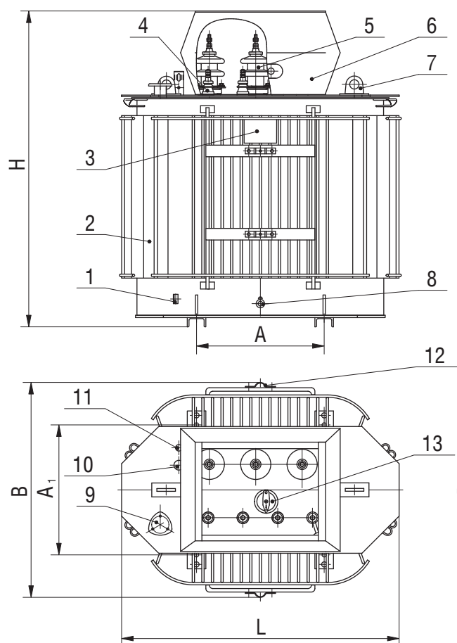
ТМЭГ - 40...250 кВ·А
